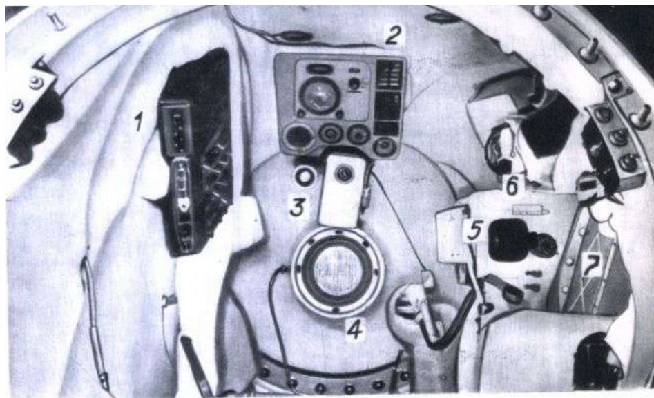
Кабина, в которой летел Юрий Гагарин: 1 — пульт пилота; 2 — приборная доска с глобусом; 3 — телевизионная камера; 4 — иллюминатор с оптическим прибором; 5 — ручка управления ориентации корабля; 6 — радиоприемник; 7 — контейнер с пищей.
